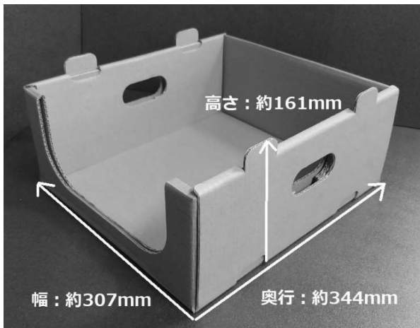
外形寸法: 幅: 約307mm × 奥行: 約344mm × 高さ: 約161mm
